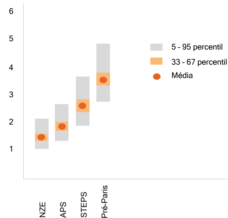
Projeção de aumento de temperatura em 2100 °C
